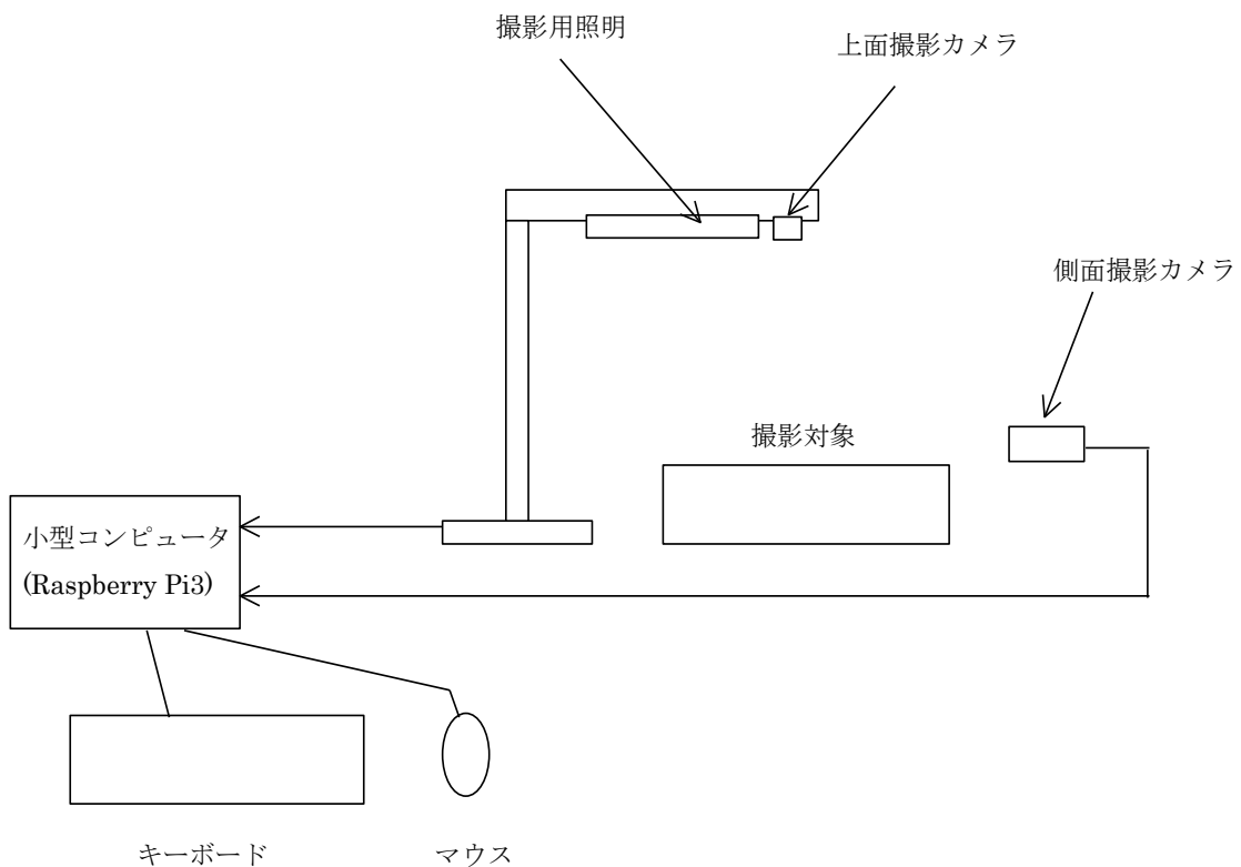
図 1 実験装置の構成[1]
